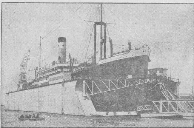
Das neue 12 000-Tonnen-Schwimmdock, das Deutschland auf Reparationskonto an Frankreich lieferte, wurde in dem nordfranzösischen Hafen Dünkirchen seiner Bestimmung übergeben.
