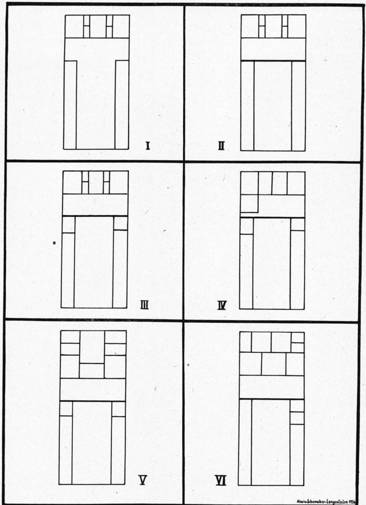
Schematische Skizzen jüngerer Grundrißveränderungen
