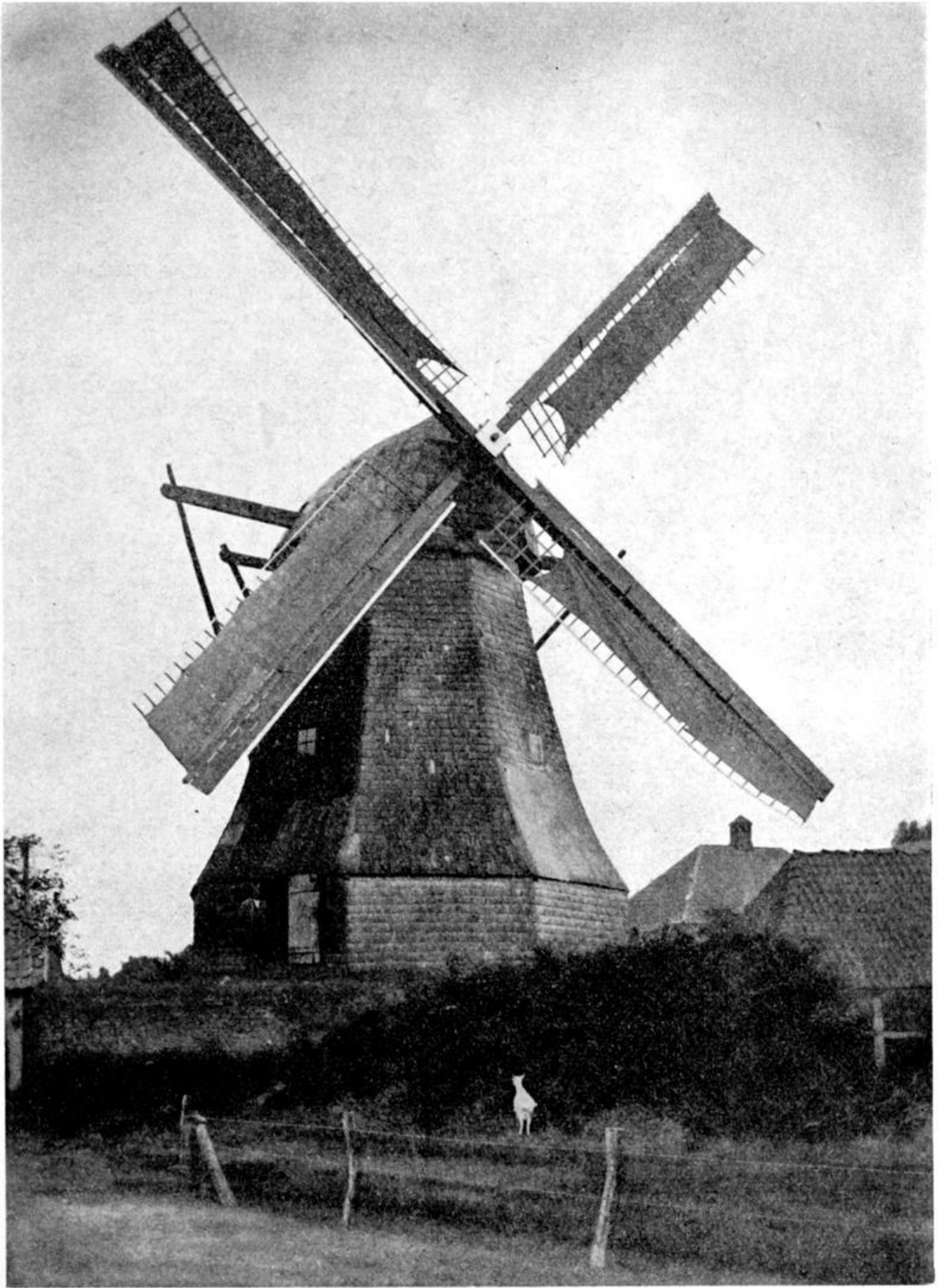
Achkantwindmühle (Erdholländer), Großenging
