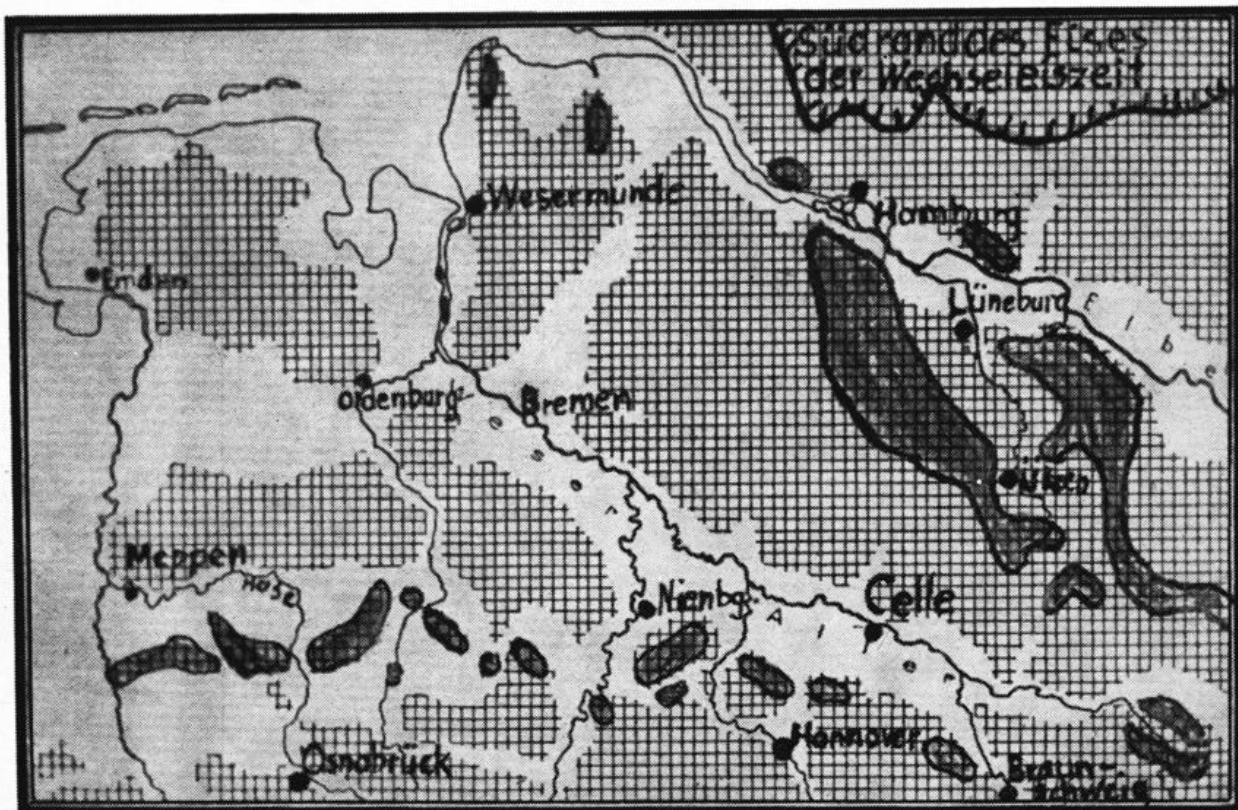
Abb. 4: Diluvialbildungen Nordwestdeutschlands (nach Hamm, Einführung in Niedersachsens Urgeschichte, 1938 — verändert), gekreuzt: allgemeine Ablagerung; schwarz: Moränen der Saalevereisung; weiß: Urstromtäler.
