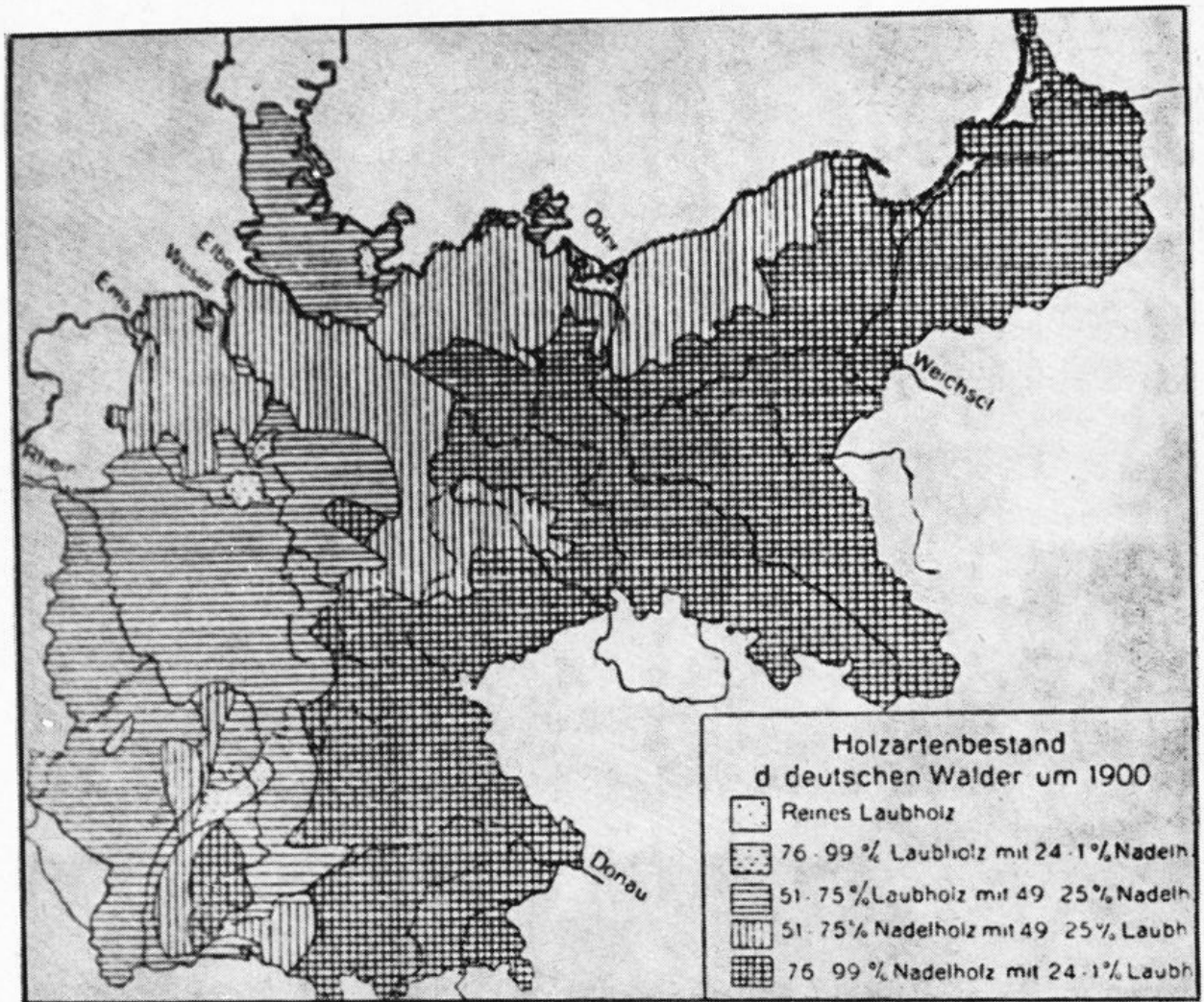
Abb. 7: Der deutsche Wald in der Gegenwart (aus Walter, Grundlagen der Pflanzenverbreitung II, 1954).
