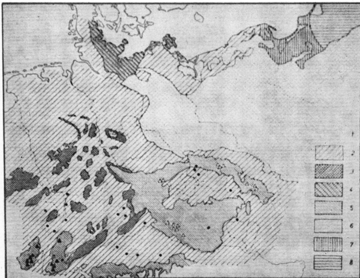
Abb. 5: Der deutsche Wald am Beginn der geschichtlichen Zeit (aus Walter, Grundlagen der Pflanzenverbreitung II, 1954).
