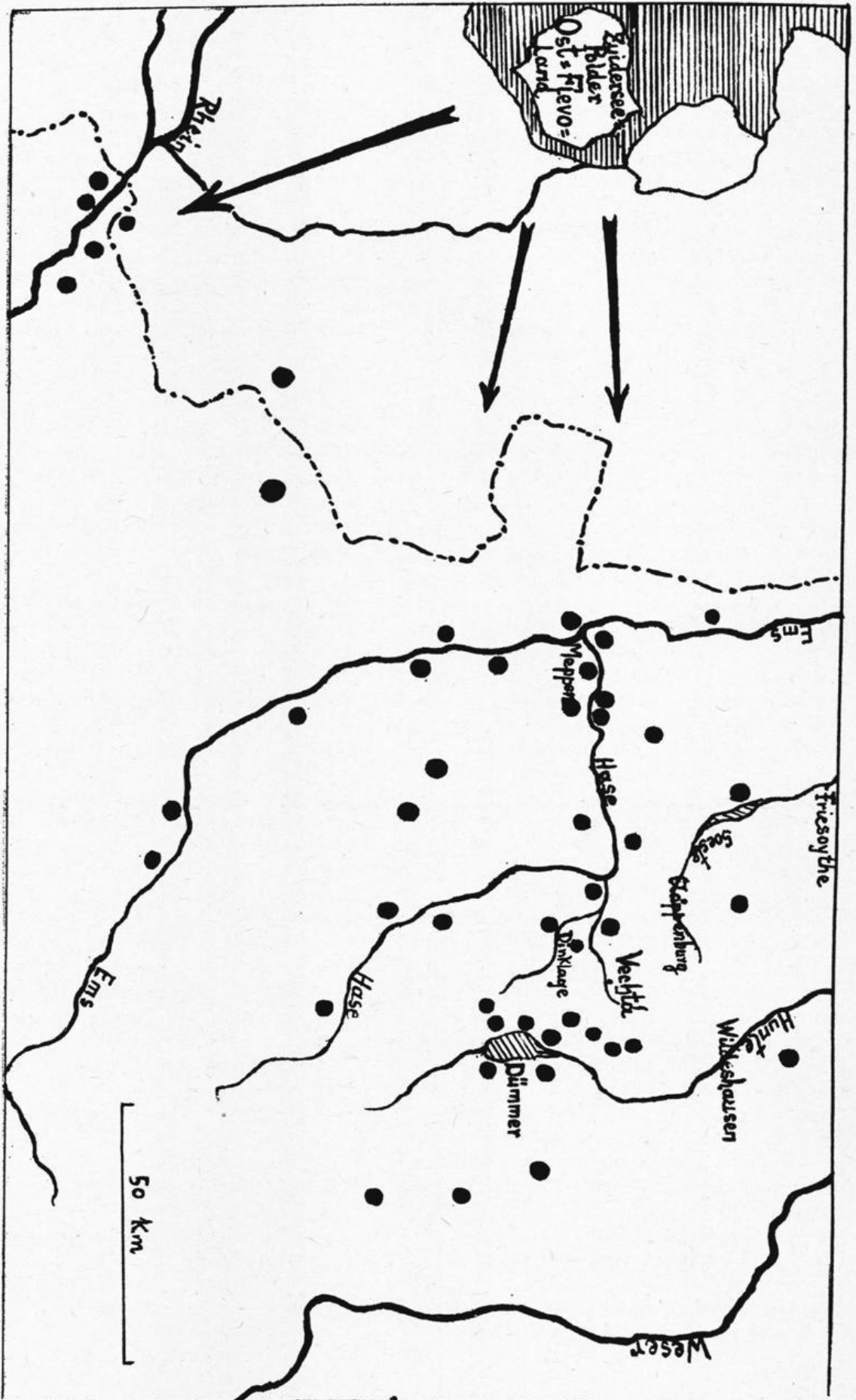
Fundorte von Moor-Kreuzkraut 1959/60 in Nordwestdeutschland, anscheinend sind die Samen vom neuen Zuidersee-Polder „Ost-Flevoland (Niederlande) aus in unsere Heimat „eingeflogen“ (J. Hürkamp).
