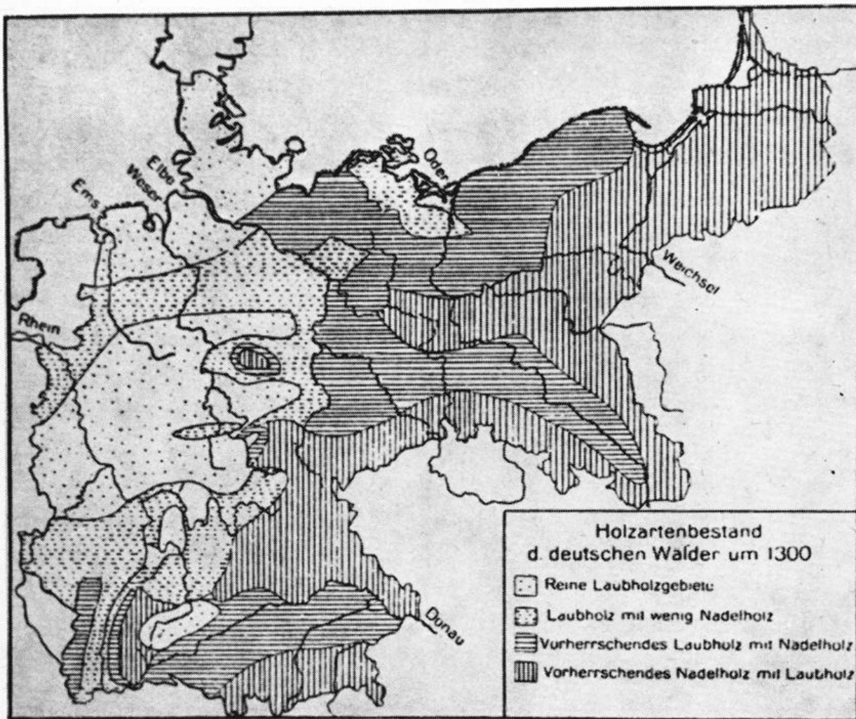
Abb. 6: Der deutsche Wald im Mittelalter (aus Walter, Grundlagen der Pflanzenverbreitung II, 1954)
