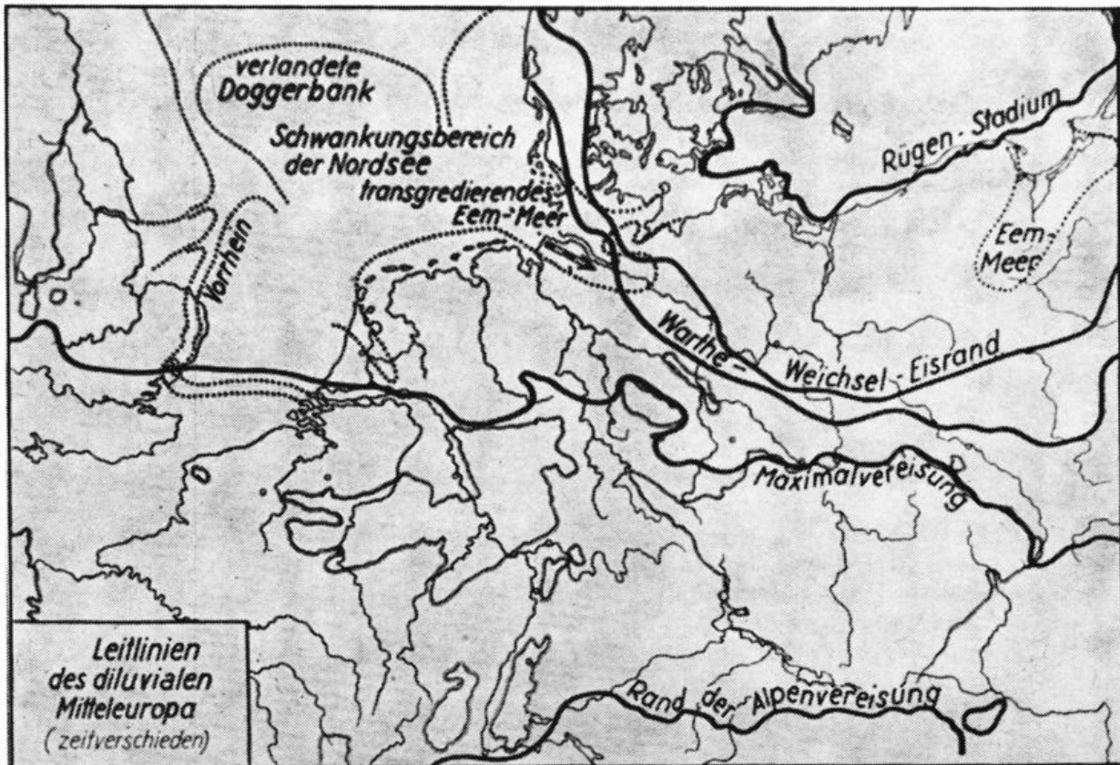
Abb. 3: Leitlinien zum deutschen Diluvium (aus Schmidt, Geologie II, 1949),
