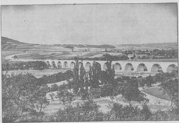
In einer Höhe von 20 Meter über der Talsohle freuht die 750 Meter lange neue Saaletalbrücke der Reichsautobahn zu schöne Tal bei Gölzig. Sie ist der Ausgangspunkt des jetzt eröffneten Streckenabschnitts der Reichsautobahn Dresden-Frankfurt a. M. Das eindrucksvolle Bauwerk, zu dem 46 000 Tonnen Werkstein benötigt wurden, besitzt 17 Öffnungen mit Halbkreisbögen in einer Spannweite von 26 bis 32 Meter je Bogen. (Sperl Bilderdienst, Zander-Multipler-R.)
