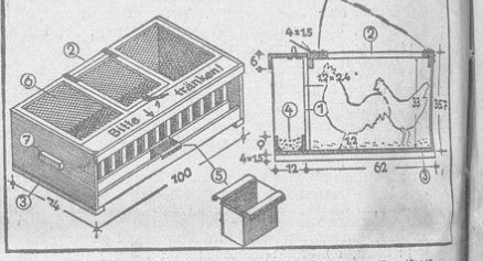
(1 = Holzleisten, 12x24 mm stark, Abstände 50 mm, 2 = Klapptür mit 2 Schenkelchen und Ueberfallverschluß, 3 = zwei Bodenleisten 15x40 mm stark, 4 = Futterrinne, in den Enden Dreieckseisen, 5 = Zinkblechbehälter, 6 = verzinktes Drahtgeflecht, 7 = Traggitter.)
