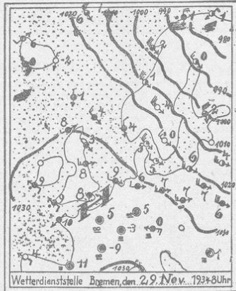
Die angegebenen Linien bedeuten: Isobaren, die die Luftdruckverhältnisse an den Beobachtungspunkten zeigen. Die Luftdruckverhältnisse an den Beobachtungspunkten sind: 1. Nebel, 2. Wolken, 3. Regen, 4. Schnee, 5. Dunst, 6. Nebel, 7. Gewitter, 8. still, 9. sehr leicht, 10. leicht, 11. schwach, 12. mäßig, 13. frisch, 14. stark, 15. sehr stark, 16. Orkan, 17. voller Sturm. Die Pfeile zeigen mit dem Winde.
